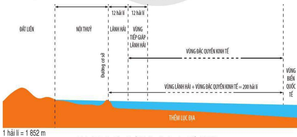
Hình 11.2. Sơ đồ mặt cắt khái quát các vùng biển Việt Nam
